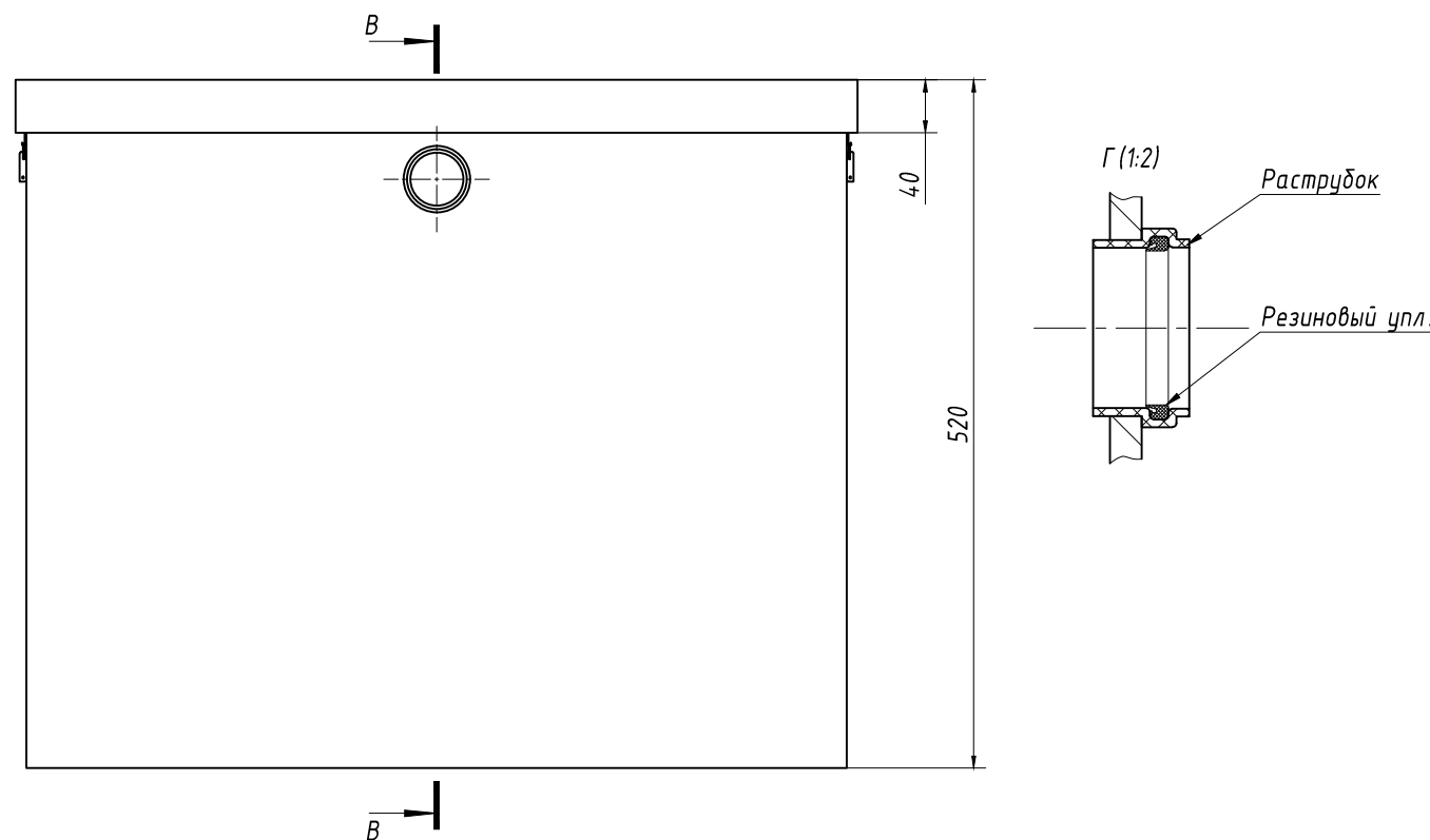
Вид Б
