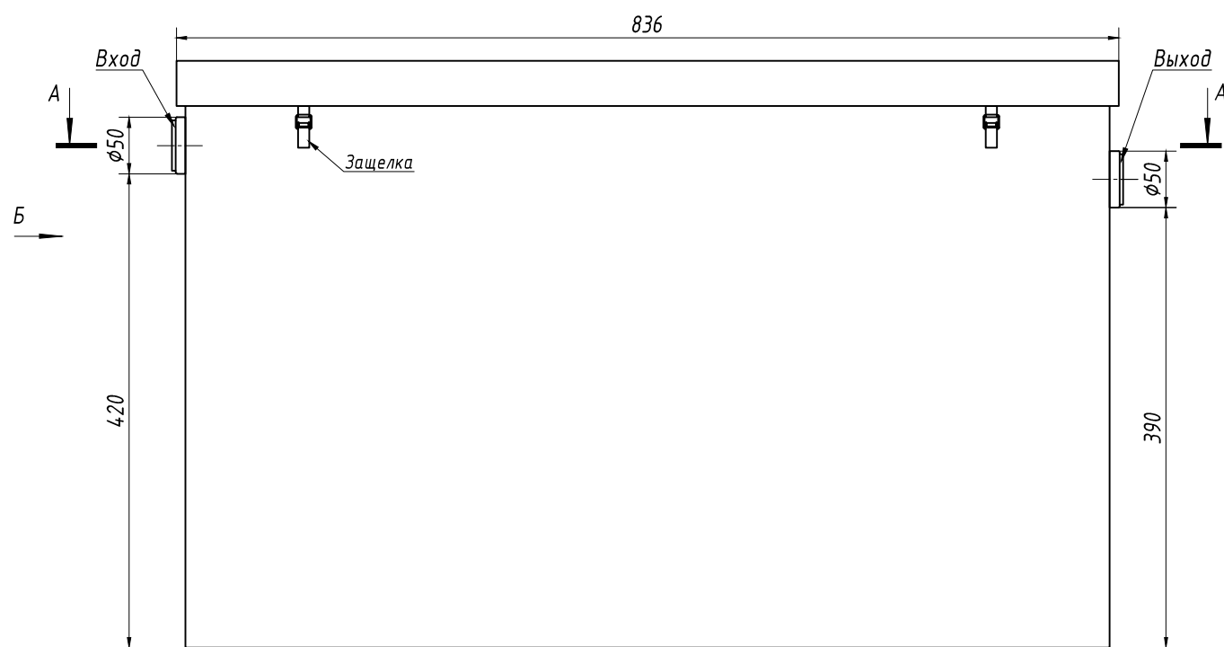
Вид спереди
